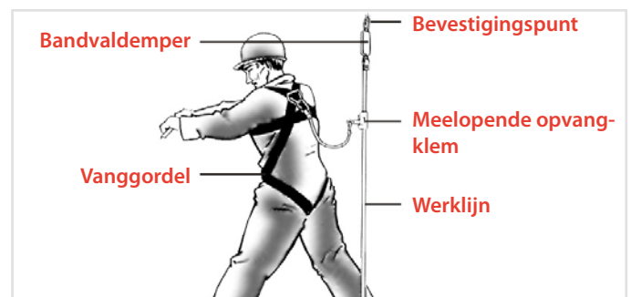
Harnas met meelopende opvangklem aan werklijn
