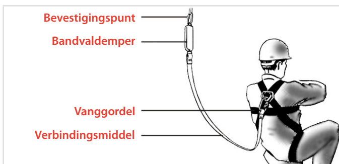
Harnas met verbindingsmiddel en bandvaldemper
